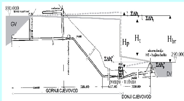
Shema padova i pritisaka hidrauličkog sistema turbina - pumpa na primjeru RHE Bajina Bašta
